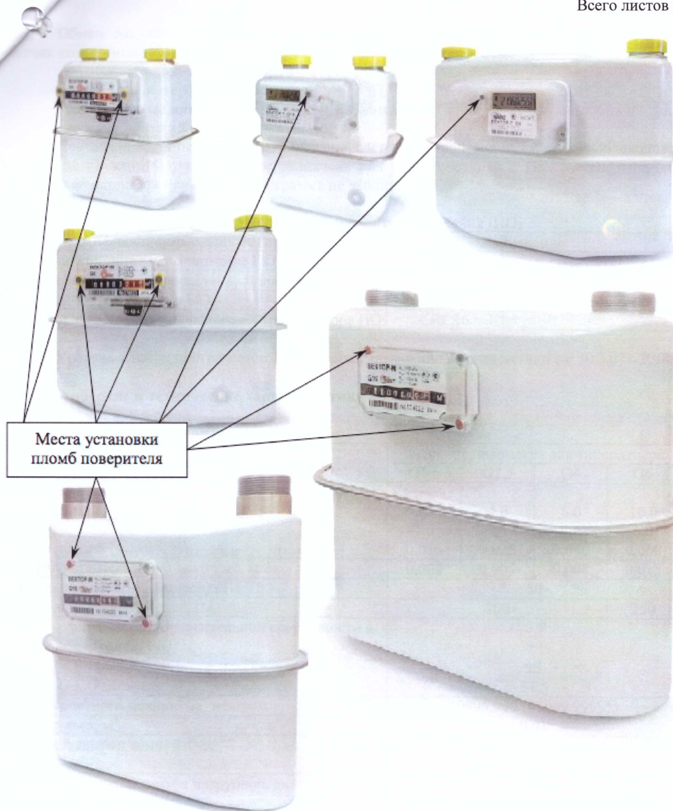
Рисунок 1 - Общий вид счетчиков газа объемных диафрагменных ВЕКТОР-М/Т
